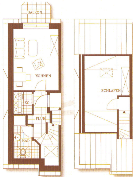
WOHNUNG 4 UND 5
